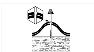
Vleugels ruimen het gat in de golfplaat op voor werking bij temperatuursverschillen.
