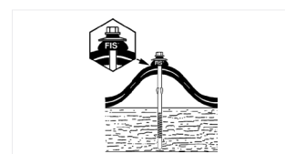
Sluitschelp zorgt voor spanningsvrije en waterdichte bevestiging.
